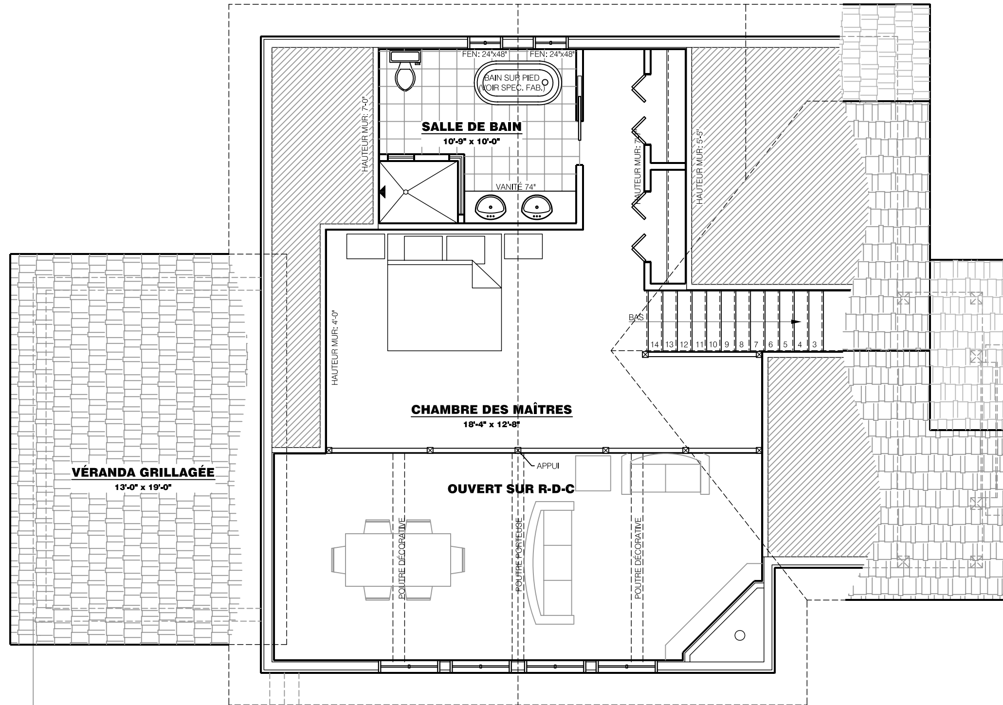
PLAN DE L'ÉTAGE Superficie habitable: 507 PiCa
