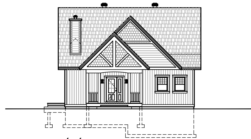
ÉLÉVATION DROITE
